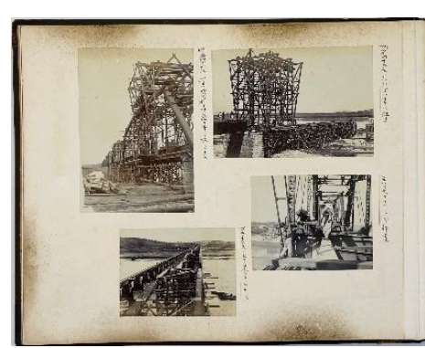
潜水函沈下準備工事之全景・工事風景・原動力工場汽缶・大洪水後之景・鋼桁組立作業／他
